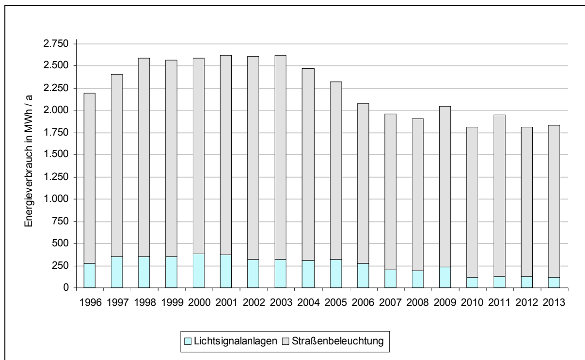
Abb. 4-17: Entwicklung des jährlichen Strombezugs (Strom - LKP) der Lichtsignalanlagen bzw. der Straßenbeleuchtung der Stadt Memmingen
