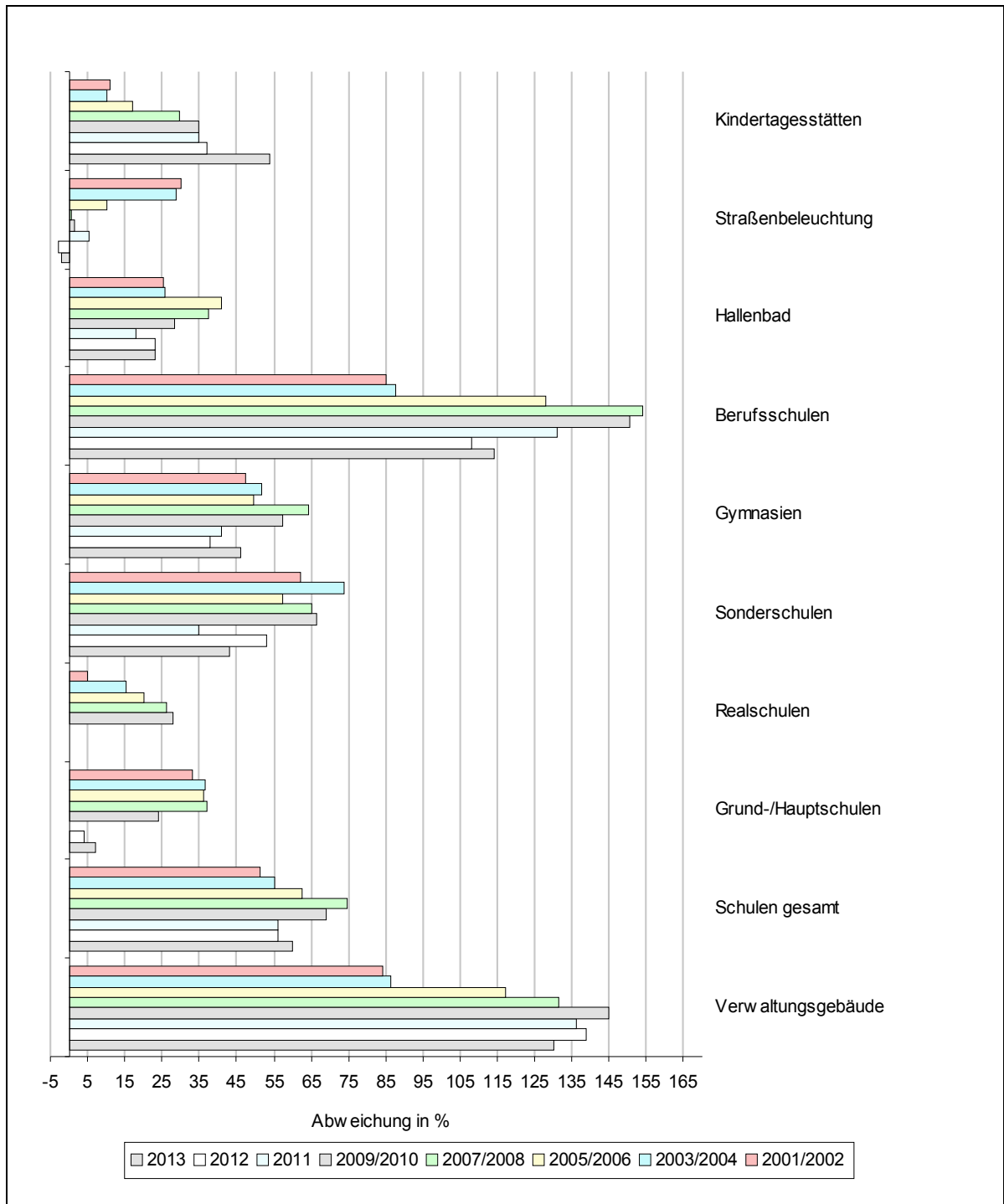
Abb. 4-24: Abweichung der Stromverbrauchskennwerte 2001 bis 2013 vom Sollwert (Modalwert ages GmbH) ausgewählter kommunaler Einrichtungen der Stadt Memmingen
