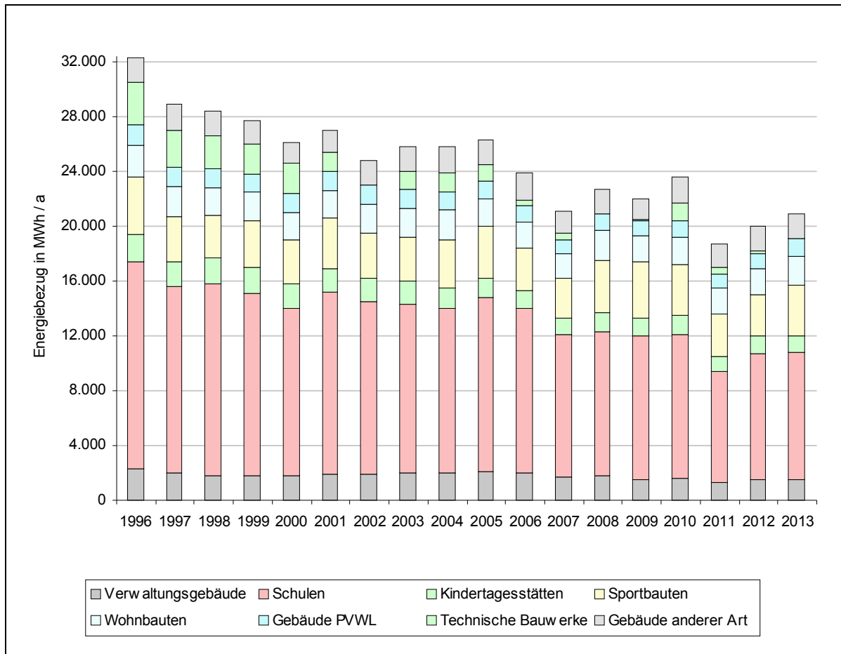
Abb. 4-27: Entwicklung des jährlichen Heizenergiebezugs der kommunalen Einrichtungen der Stadt Memmingen nach Gebäude- bzw. Anlagengruppen
