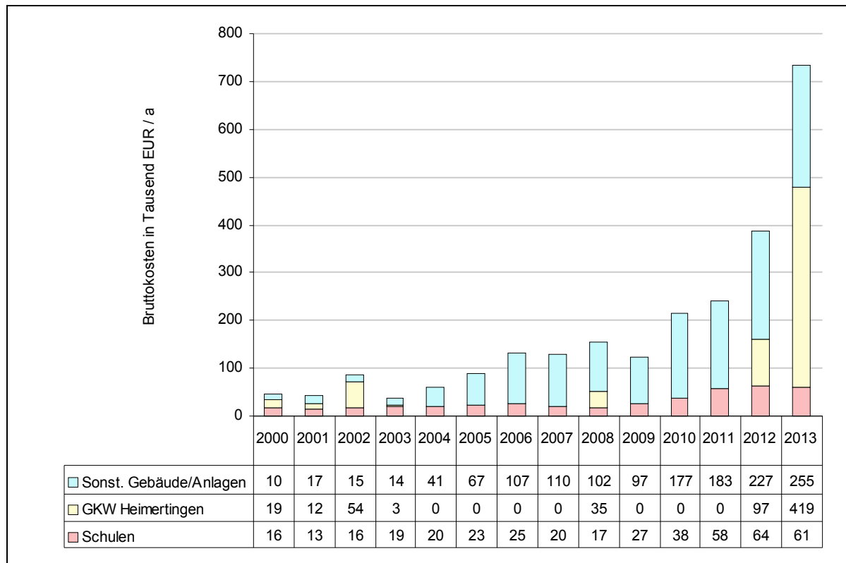
Abb. 4-26 Vermiedene Kosten für Fremd- und Eigenstrom bei der Stadt Memmingen 2000 bis 2013
