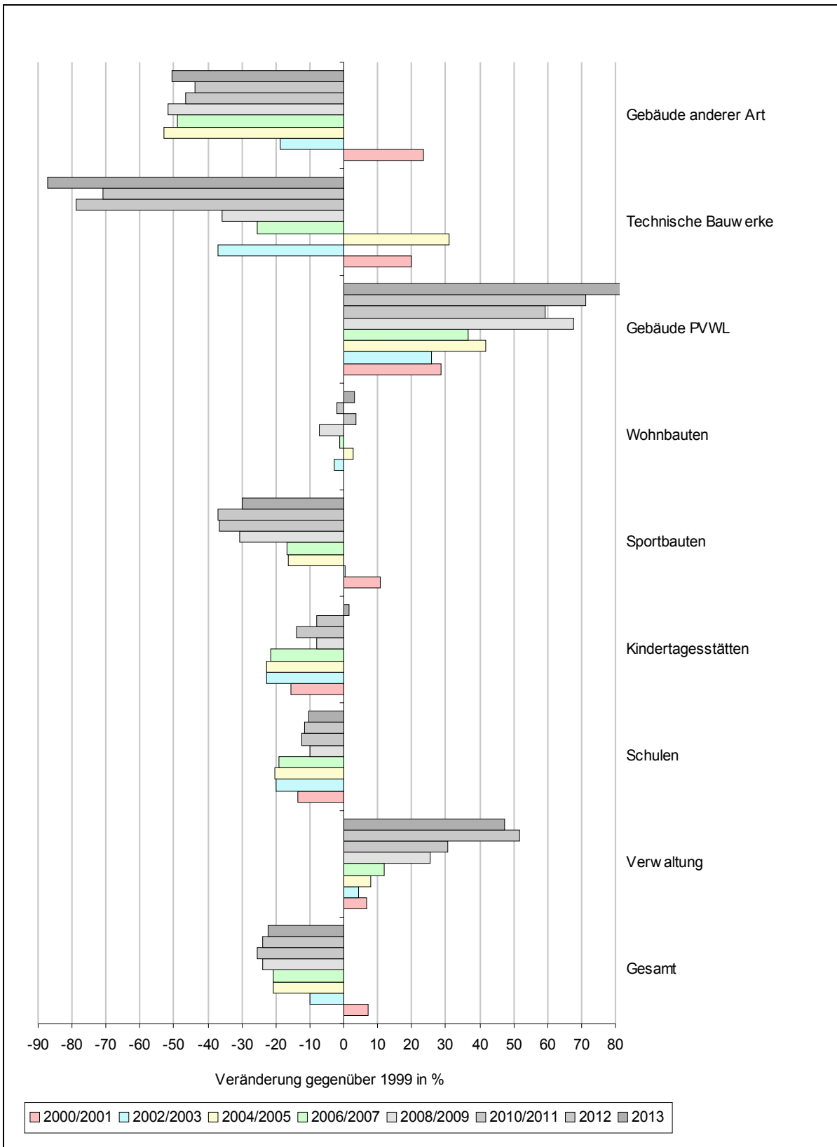
Abb. 4-40: Veränderungen des Trinkwasserverbrauchs kommunaler Einrichtungen der Stadt Memmingen im Vergleich zu 1999 nach Gebäudegruppen
