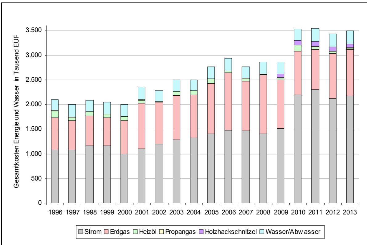
Abb. 1-5 Zeitliche Entwicklung der Kosten für Energie- und Trinkwasserbezug sowie Entwässerung 1996 bis 2013
