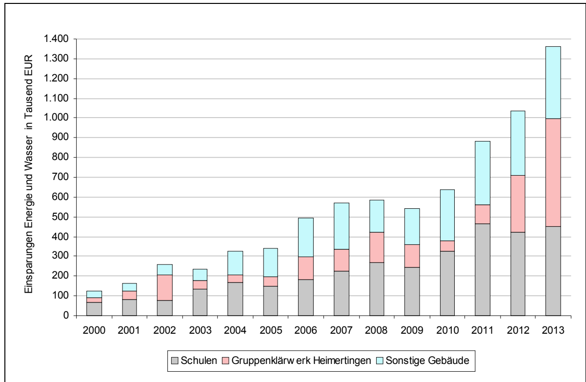
Abb. 4-7: Vermiedene Kosten (Brutto) der kommunalen Einrichtungen der Stadt Memmingen nach »Bereichen«
