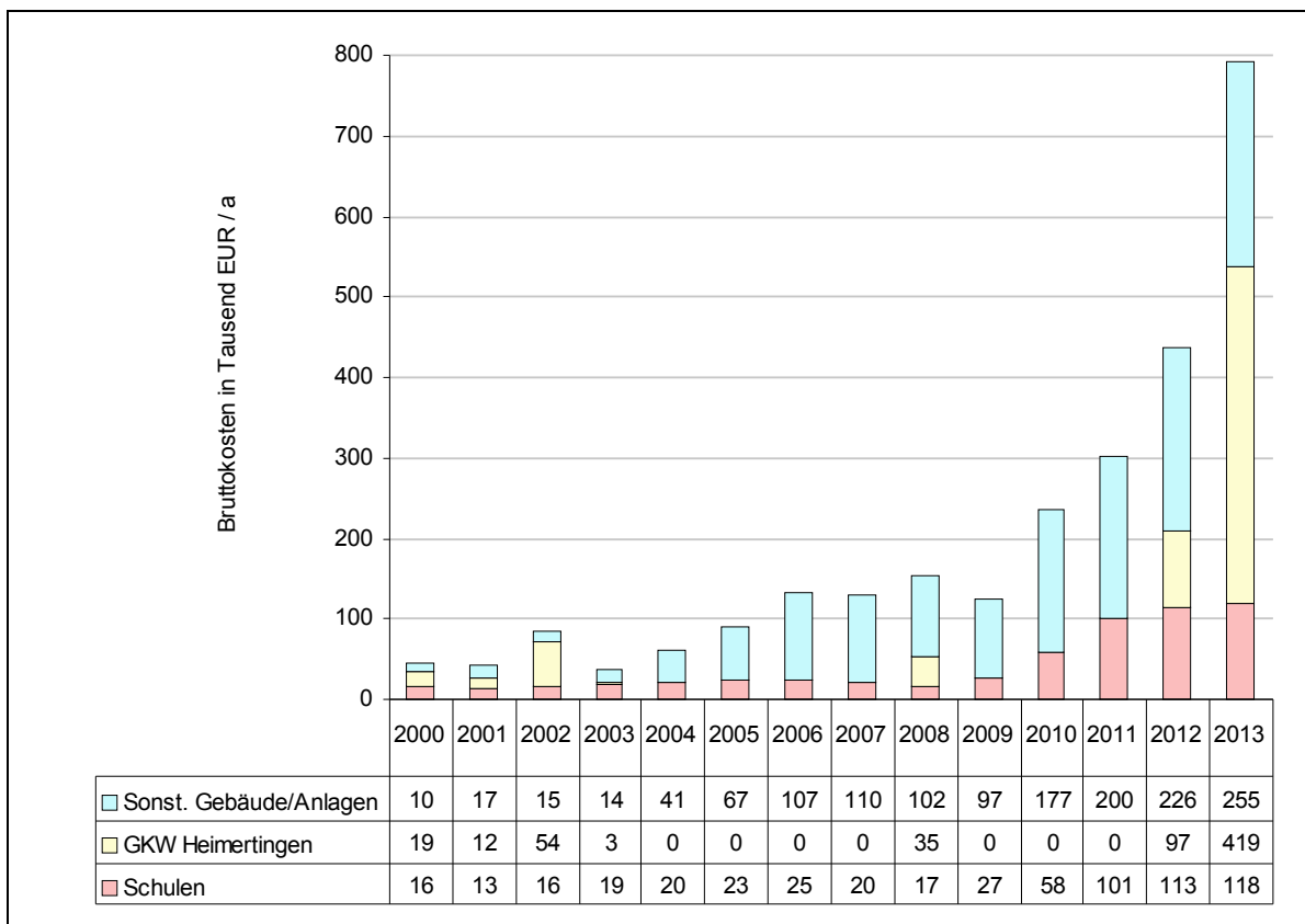
Abb. 4-25 Vermiedene Kosten für Fremdstrom bei der Stadt Memmingen 2000 bis 2013
