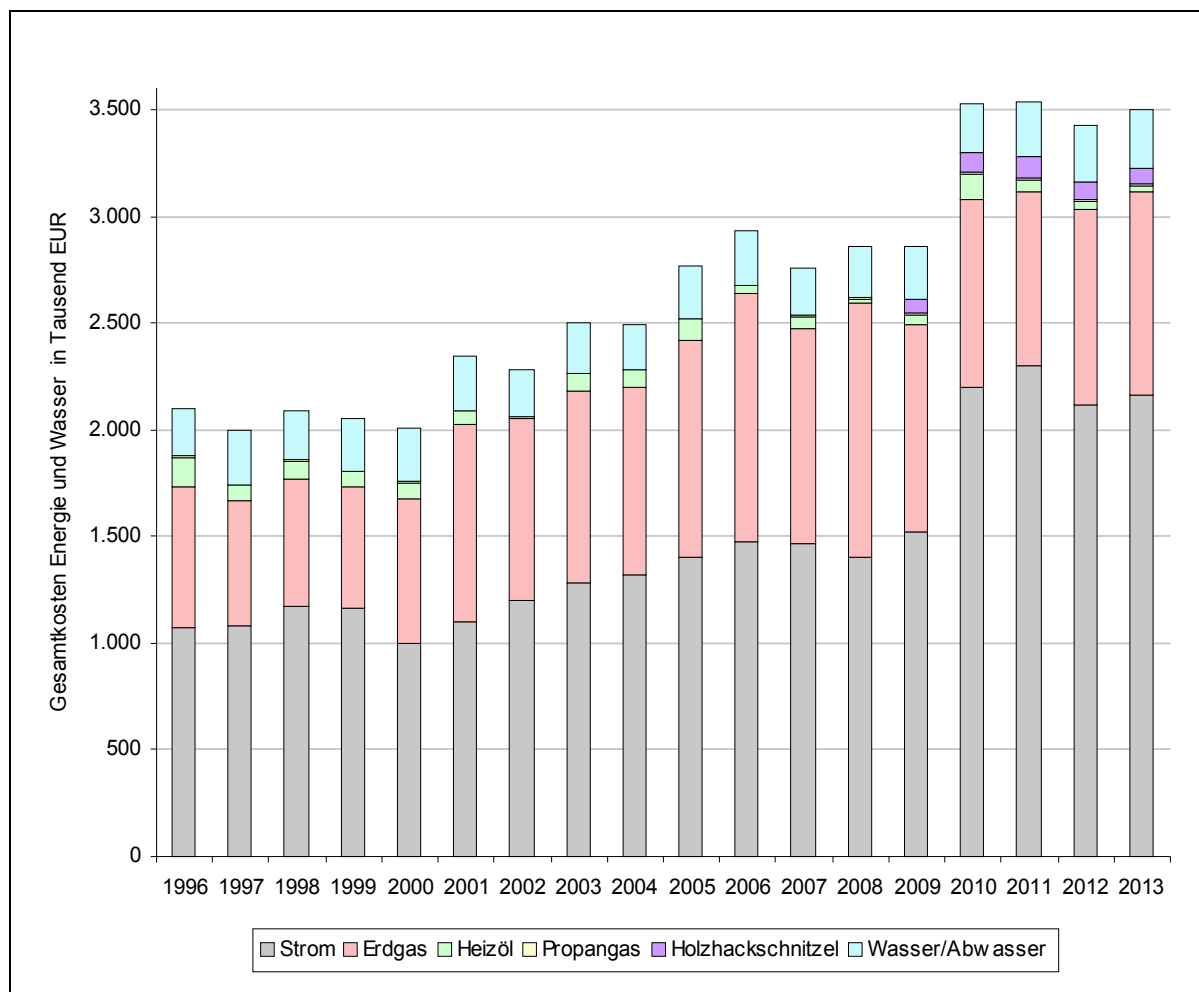
Abb. 4-3: Entwicklung der Energie- und Wasserkosten (Brutto) der kommunalen Einrichtungen der Stadt Memmingen nach Energieträgern
