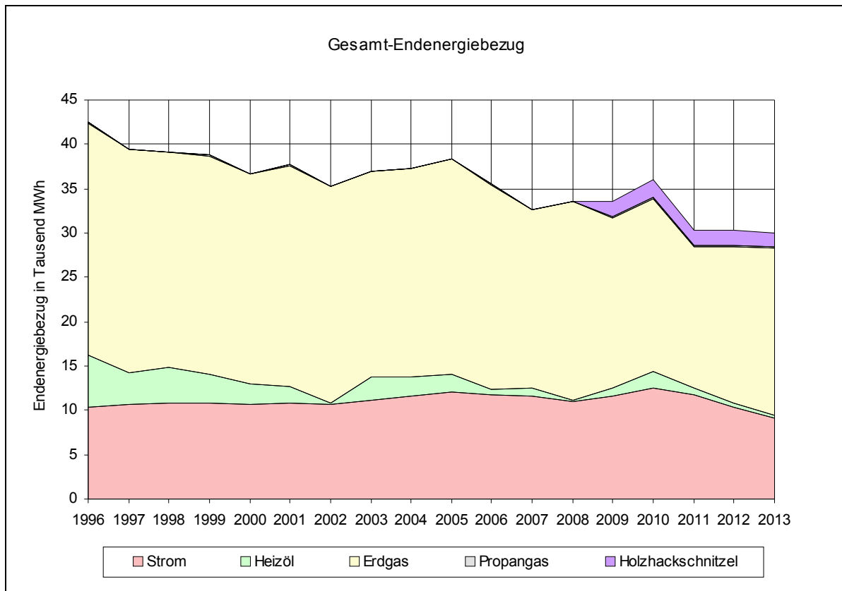
Abb. 1-1 Zeitliche Entwicklung des Endenergiebezugs 1996 bis 2013 nach Energieträgern
