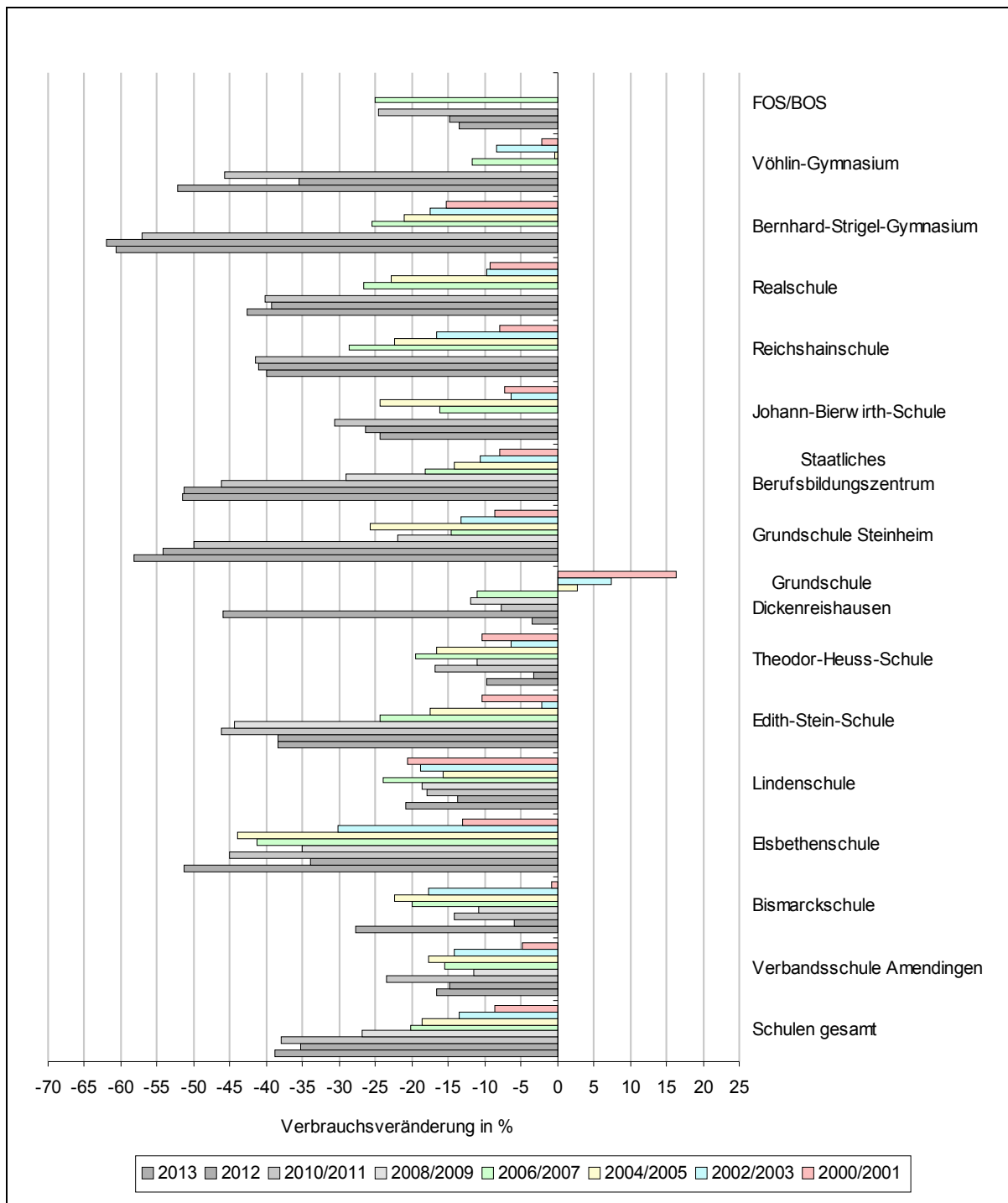
Abb. 4-30: Klimabereinigte Heizenergiebezugsänderungen der Schulen der Stadt Memmingen gegenüber dem Referenzwert
