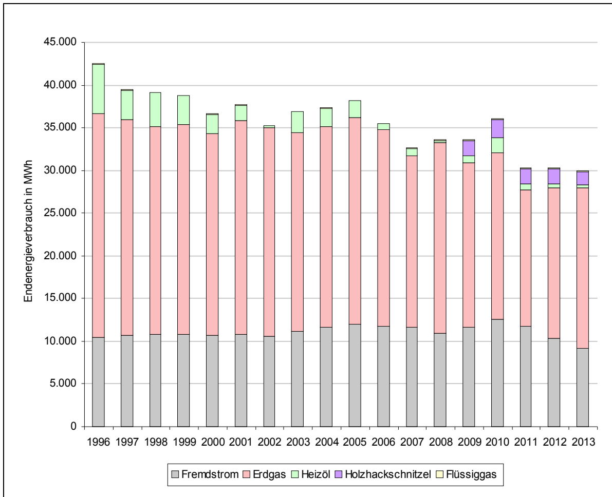
Abb. 4-9: Entwicklung des Endenergiebezugs der kommunalen Einrichtungen der Stadt Memmingen nach Energieträgern
